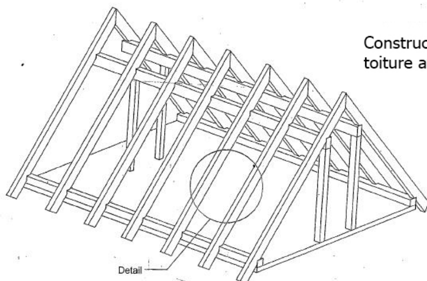
Détail
