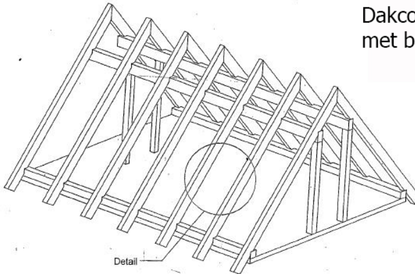
Detail Installatie van de nageldichtband
